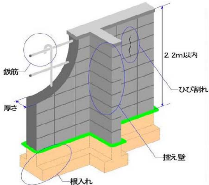
ブロック塀のチェック項目
