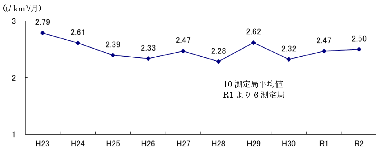
図3 降下ばいじん量年度別推移
