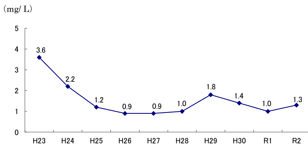
図 12 BOD年度別推移 吉和川上流（高頭）
