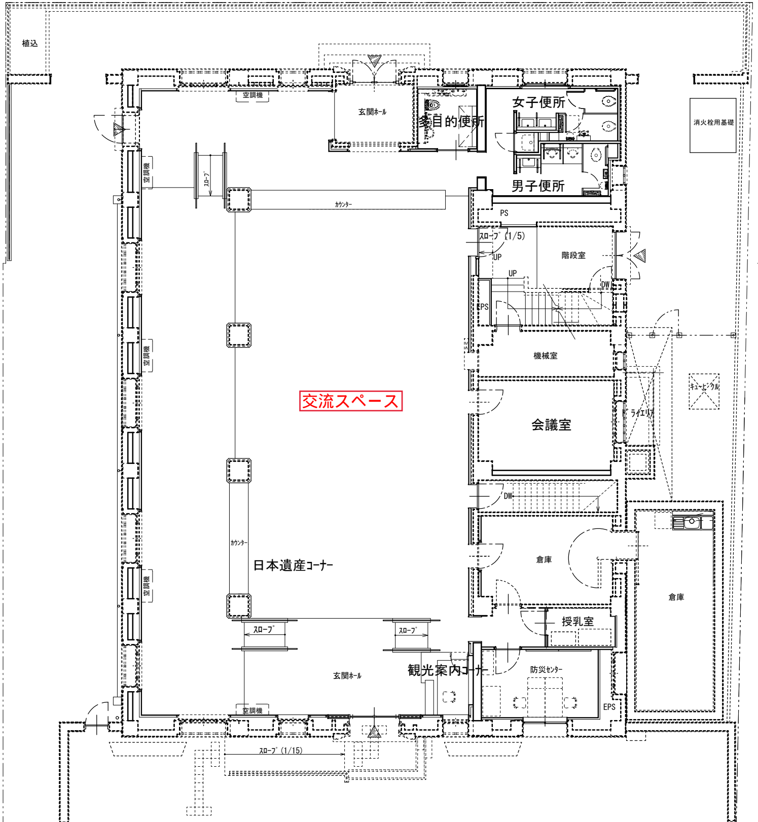
1階平面図
