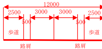
横断面 (改良後)
