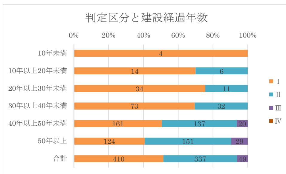
図 1-8 判定区分と建設経過年数
