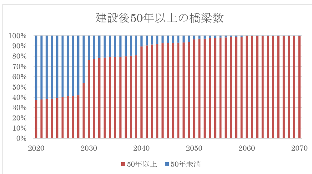
図 1-2 建設後 50 年以上の橋梁数
