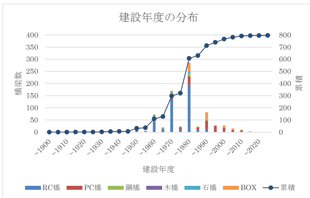
図 1-1 建設年度の分布
