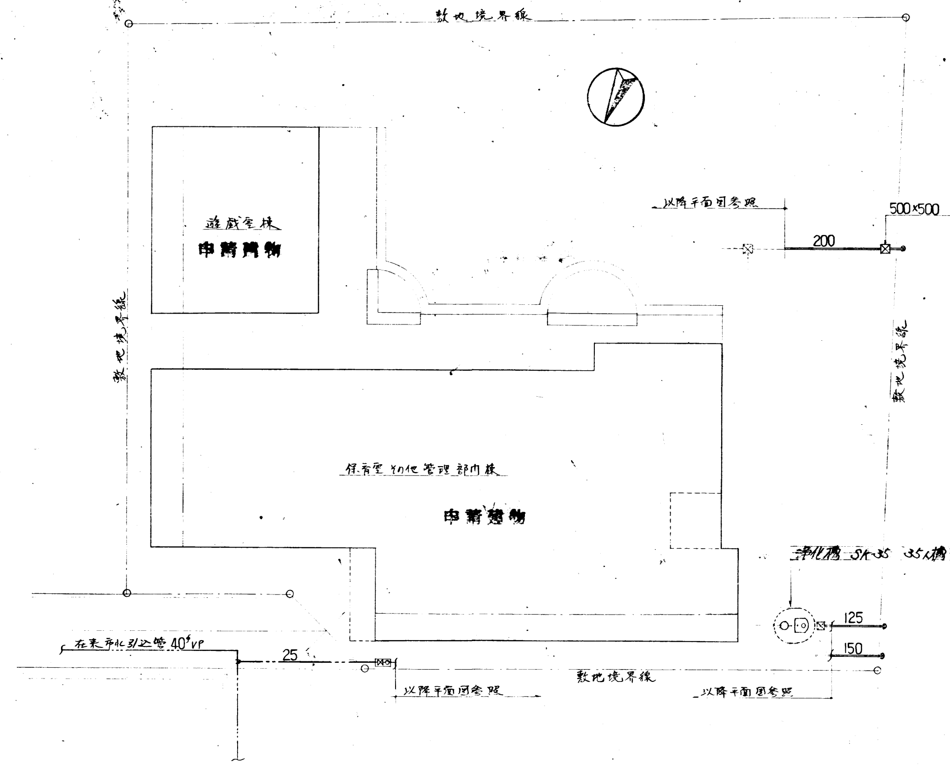
配置図 縮尺: 1:200
