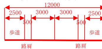
横断図（改良後）
