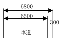
横断図（現況）
