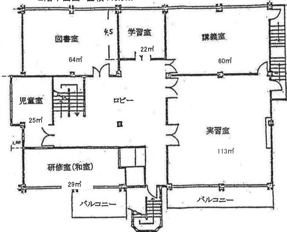
2階平面図 面積445.5㎡
